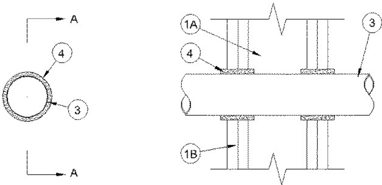
Section A-A
